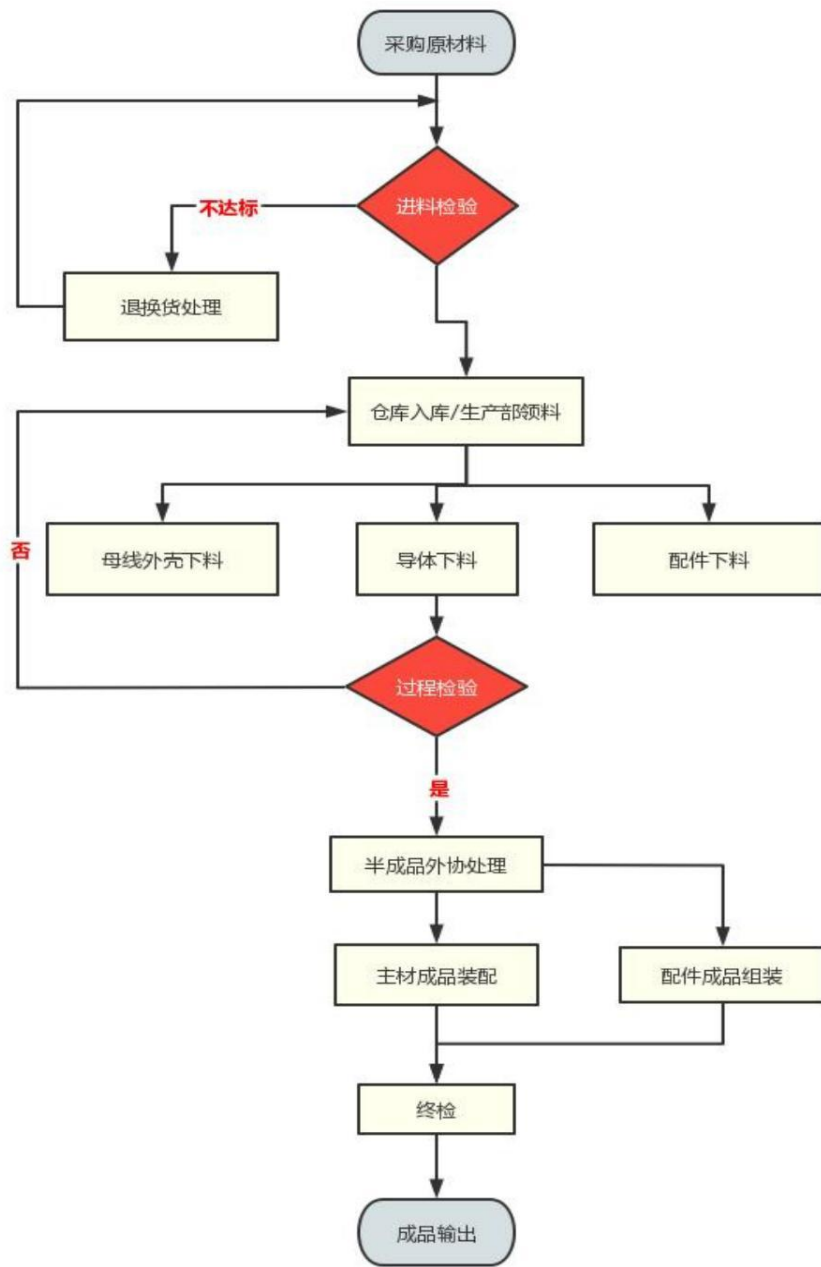
图 2.2 工艺流程图
